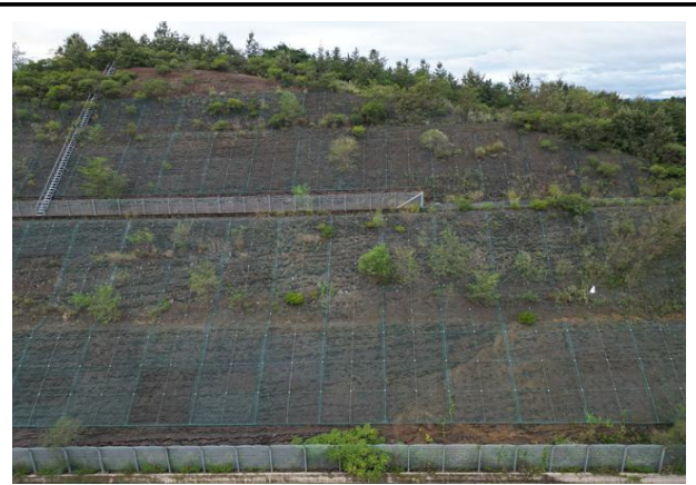
낙석방지망 전경
